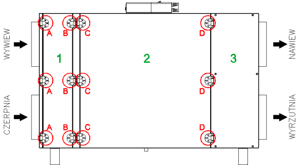
Rys.1. Panele inspekcyjne oraz zawiasy klamrowe urządzenia AirPack 1450
