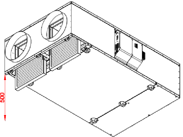
Rys.2. Demontaż filtrów
