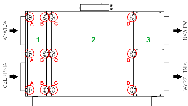
Rys.1. Panele inspekcyjne oraz zawiasy klamrowe urządzenia AirPack 1700
