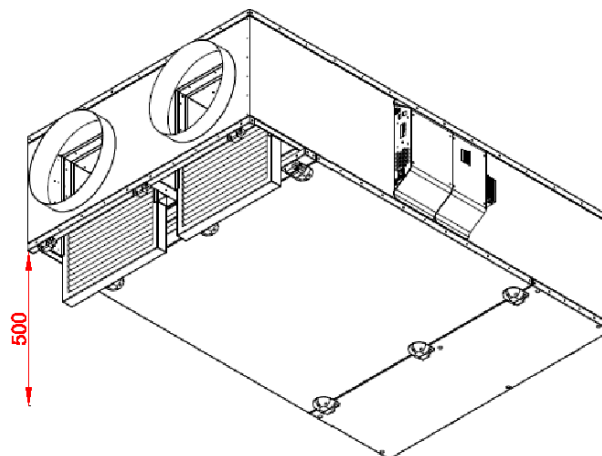
Rys.2. Demontaż filtrów
