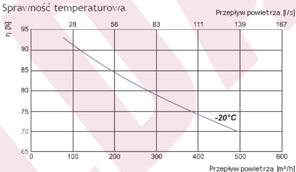
Sprawność temperaturowa
